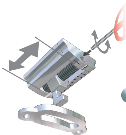
Großer, sagittaler Verstellweg von 7 mm
